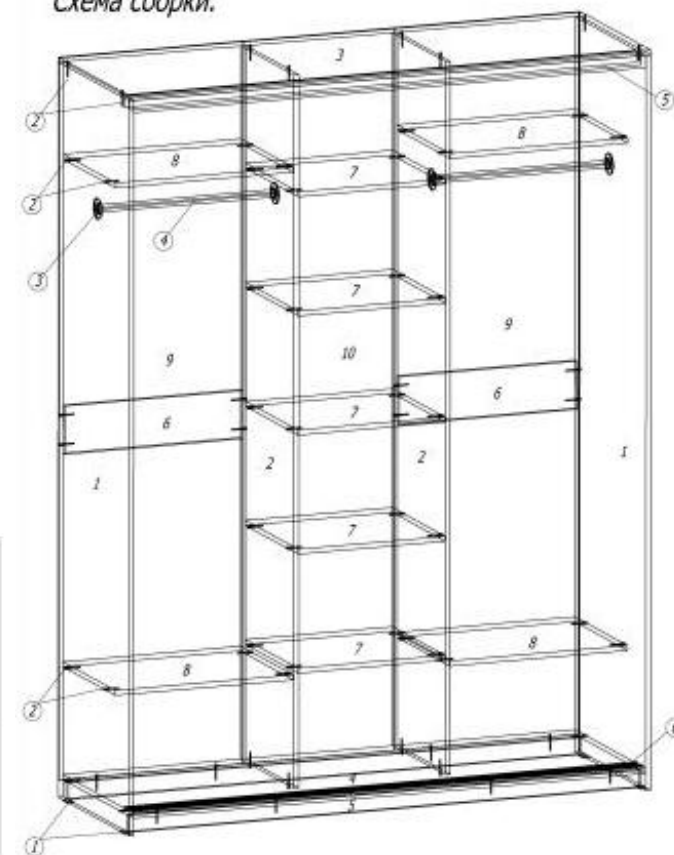
Схема сборки.
